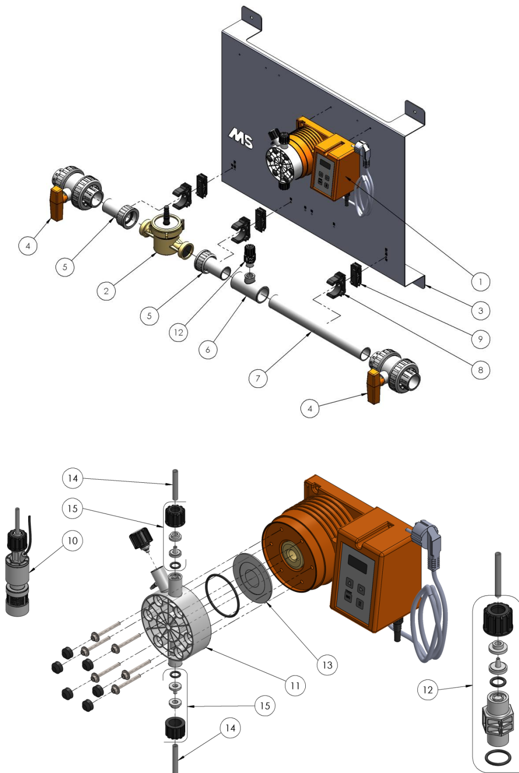
Abb. 1.1 Explosionszeichnung
